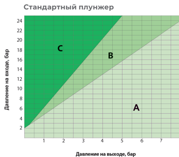
Кавитационный график
